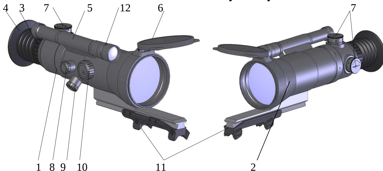
Рис. 1 Прибор «Dedal-470-xxx(110)»
